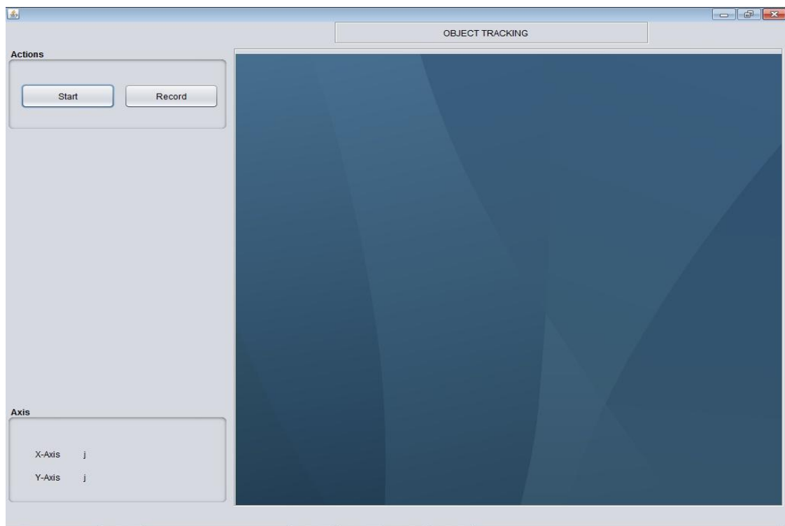
Fig.3 Tracking Module
