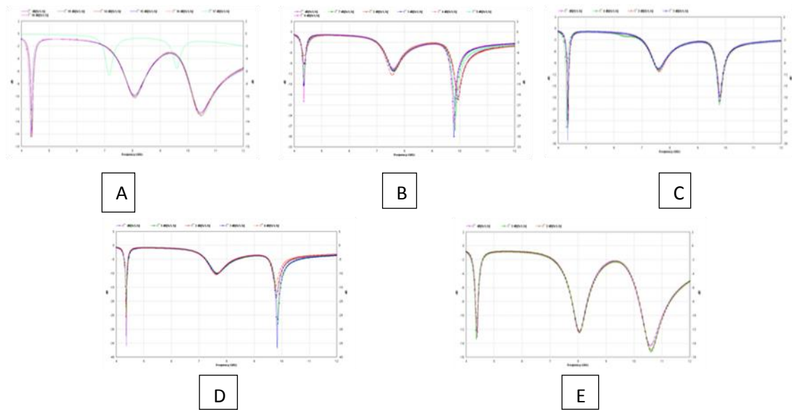
Fig.15: Simulated S11 curves for Tripe band antenna (A) Diode D1, D2 and D3 (B) Diode D2, D3 and D4 (C) Diode D3, D4 and D5 (D) Diode D4, D5 and D1 (E) Diode D5, D1 and D2
