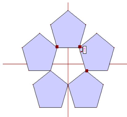
Fig.12. Diodes D4, D5 and D1 embedded in patch
