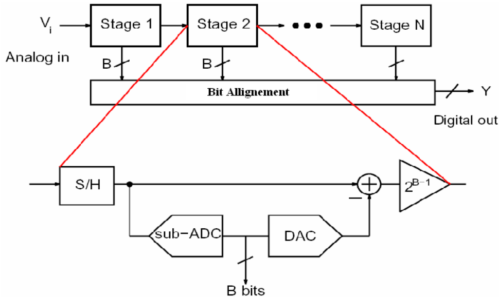
Figure.1BlockdiagramofapipelinedADC
